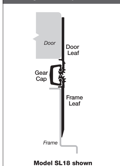
Fig. 3 Door Open 180°
