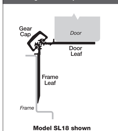
Fig. 2 Door Open 90°
